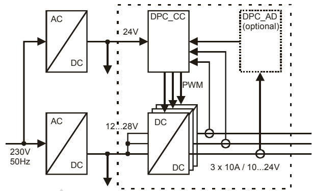
Fig. 3.4.5.1: Converter concept 3*10A.
