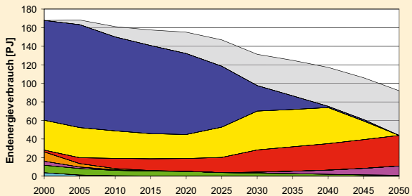
■ Widerstandsheizung elektrisch ■ Biomasse ■ Fernwärme ■ Sparmassnahmen * ■ Wärmepumpe elektrisch ■ Erdgas ■ Öl ■ Andere
