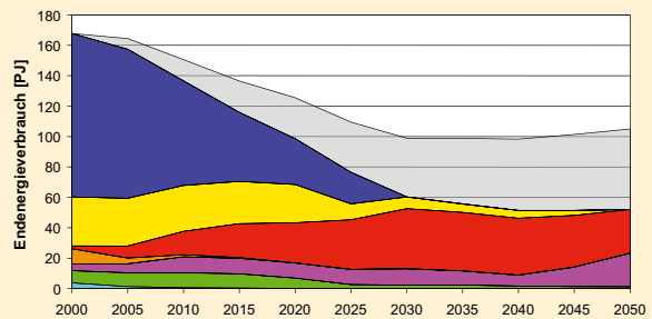
■ Widerstandsheizung elektrisch ■ Biomasse ■ Fernwärme ■ Sparmassnahmen * ■ Wärmepumpe elektrisch ■ Erdgas ■ Öl ■ Andere
