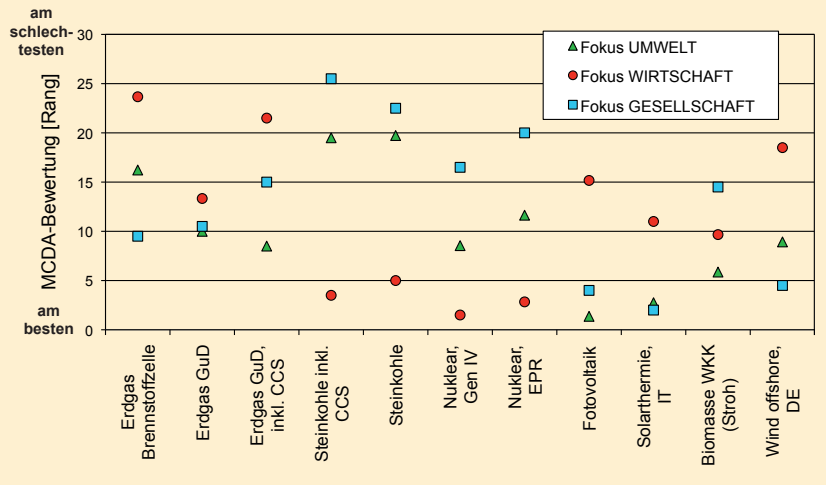
Grafik 6: Ergebnisse aus dem Projekt NEEDS: MCDA-Bewertung für die Stromversorgung der Schweiz im Jahr 2050 mit drei verschiedenen Indikatorgewichtungen, s. Grafik 7 (PSI/NEEDS; Schenler et al. 2009); Abk. s. Grafik 3 und Tabelle 2.
