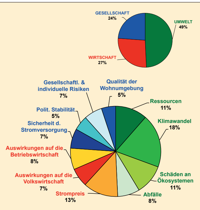
Grafik 4: Durchschnittliche Gewichtung der Indikatoren zur Technologienbewertung (PSI/NEEDS; Schenler et al. 2009), ermittelt mit einer Online-Umfrage unter Akteuren in der Energieversorgung in Europa (nicht repräsentativ für den Bevölkerungsschnitt).
