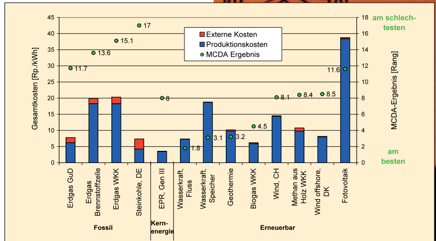
Grafik 3: Ergebnisse aus dem Projekt Nachhaltigkeitsbewertung für ein grosses Energieunternehmen. Gesamtkosten der Stromerzeugung (Säulen) vs. MCDA-Ergebnisse (Punkte) für die Versorgung der Schweiz im Jahr 2030 (Roth et al., 2009). Die Grafik zeigt eine Auswahl der insgesamt 18 bewerteten Systeme. GuD: Gas- und Dampfkraftwerk, WKK: Wärme-Kraft-Kopplung, EPR: Europäischer Druckwasserreaktor
