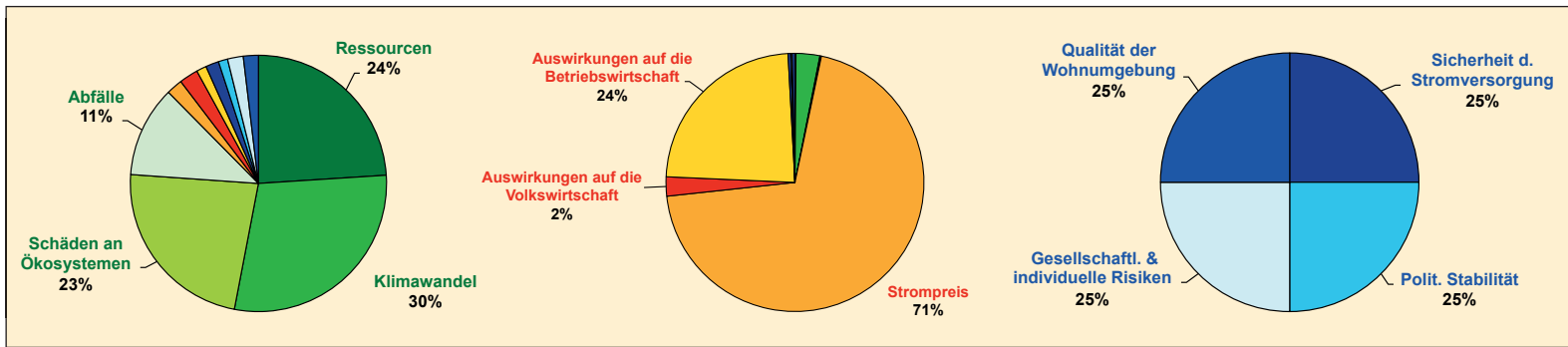
Grafik 7: Gewichtung der Indikatoren zur Technologienbewertung für sehr einseitige Gewichtungsprofile (kleine Teilmengen der befragten Akteure). Links: Schwerpunkt Umwelt, Mitte: Schwerpunkt Wirtschaft, Rechts: Schwerpunkt Gesellschaft (PSI/NEEDS; Schenler et al. 2009).
