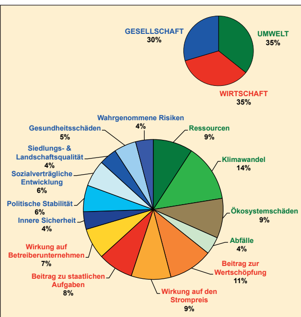
Grafik 2: Gewichtungsschema für die Indikatoren zur Technologienbewertung (Roth et al., 2009), ermittelt als Durchschnitt einer Befragung von 85 MitarbeiterInnen eines grossen Energieunternehmens (nicht repräsentativ für den Bevölkerungsschnitt).
