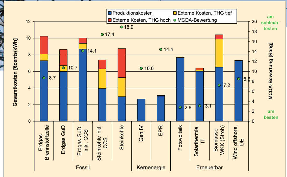
Grafik 5: Ergebnisse aus dem Projekt NEEDS: Gesamtkosten der Stromerzeugung (Säulen) vs. MCDA-Ergebnisse (Punkte) für die Versorgung der Schweiz im Jahr 2050 (PSI/NEEDS; Schenler et al. 2009). Die Grafik zeigt eine Auswahl der insgesamt 26 bewerteten Systeme. THG hoch/tief: hohe bzw. tiefe Schadenskosten durch den Klimawandel (Treibhausgasemissionen); Abk. s. Grafik 3 und Tabelle 2.
