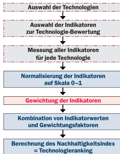
Grafik 1: Schema für den Ablauf einer Multi-Kriterien-Analyse (subjektive Elemente in rot, objektive Schritte in blau).
